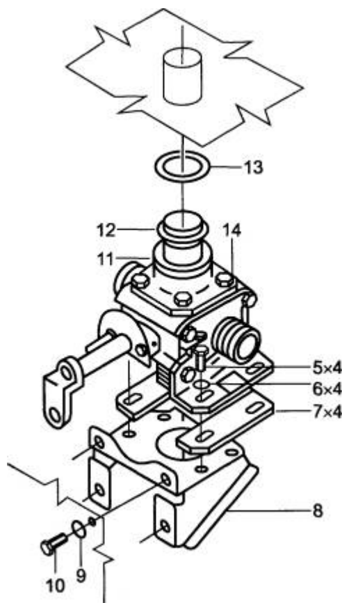
Рисунок А.1 - Пример указания количества одинаковых деталей
