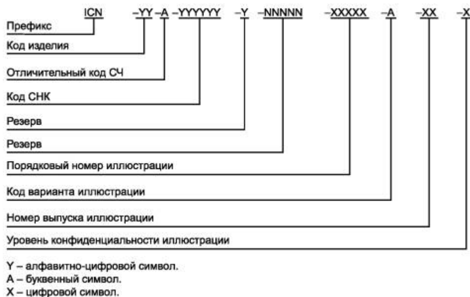
Рисунок Г.2 - Структура обозначения иллюстрации
