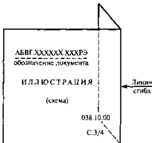
Рисунок 1 - Оформление листов увеличенного формата (правила фальцовки)
